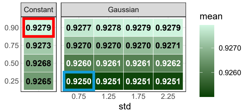
FDR
