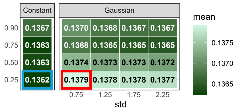
Precision
