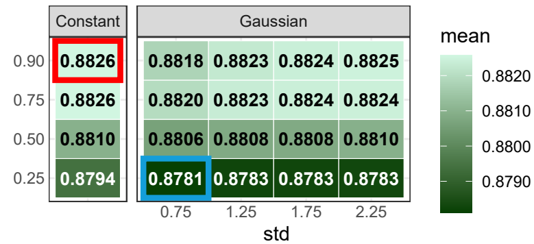
NPV
